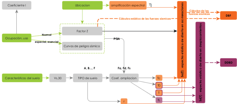
Figura 33 : Cadena de determinación de la demanda sísmica
