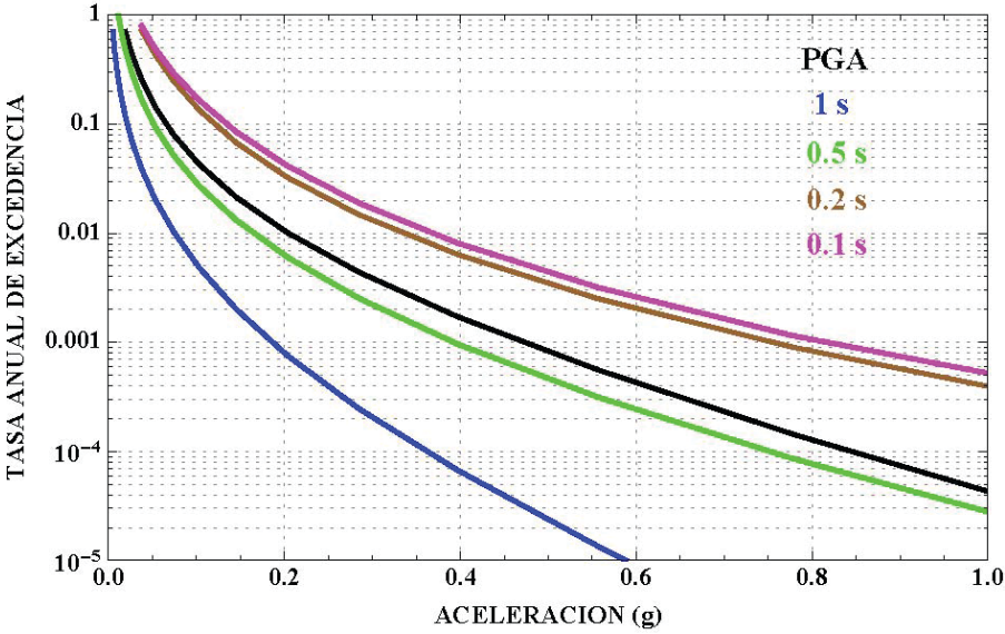
Figura 26: Curvas de peligro sismico, Machala.
