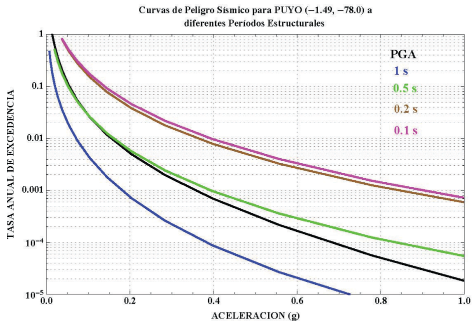
Figura 29 : Curvas de peligro sísmico, Puyo.
