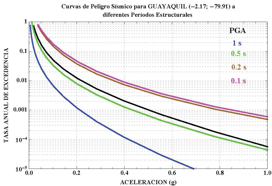
Figura 25: Curvas de peligro sísmico, Guayaquil.
