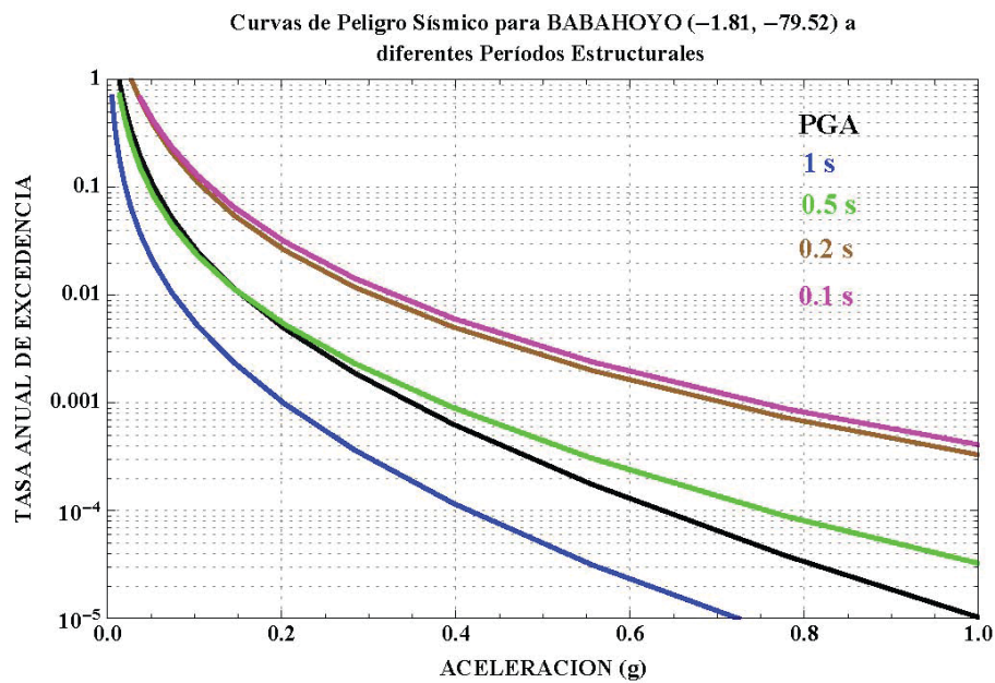
Figura 24: Curvas de peligro sísmico, Babahoyo.
