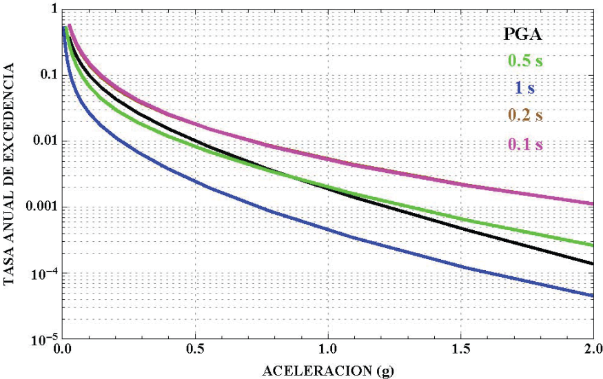
Curvas de Peligro Sísmico para ESMERALDAS (0.97; -79.65) a diferentes Periodos Estructurales
