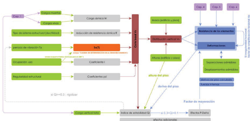
Figura 35 : esquema del diseño basado en fuerzas (DBF)
