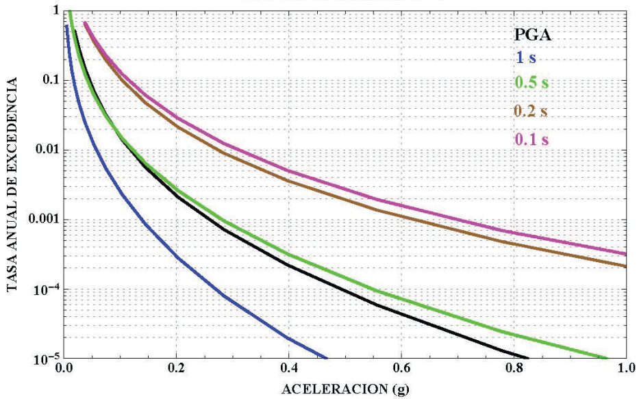
Figura 18 : Curvas de peligro sísmico, Cuenca.
