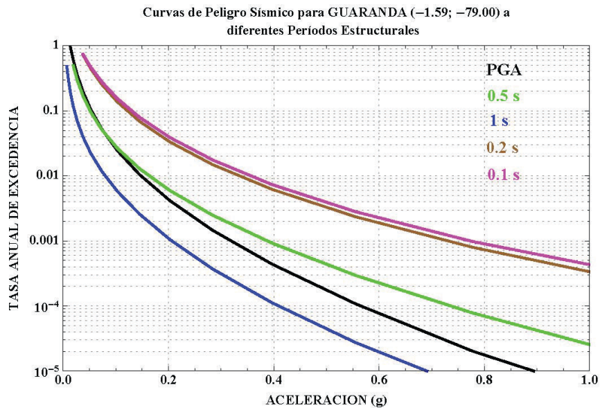
Figura 16 : Curvas de peligro sísmico, Guaranda.
