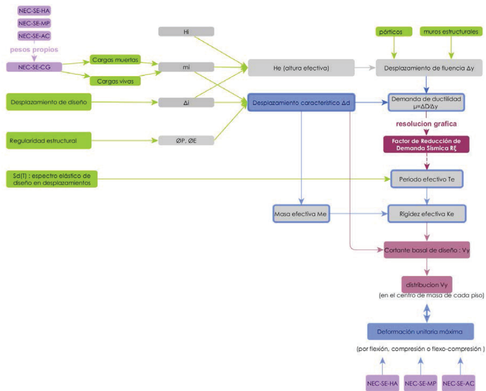
Figura 36 : Esquema del diseño basado en desplazamientos
