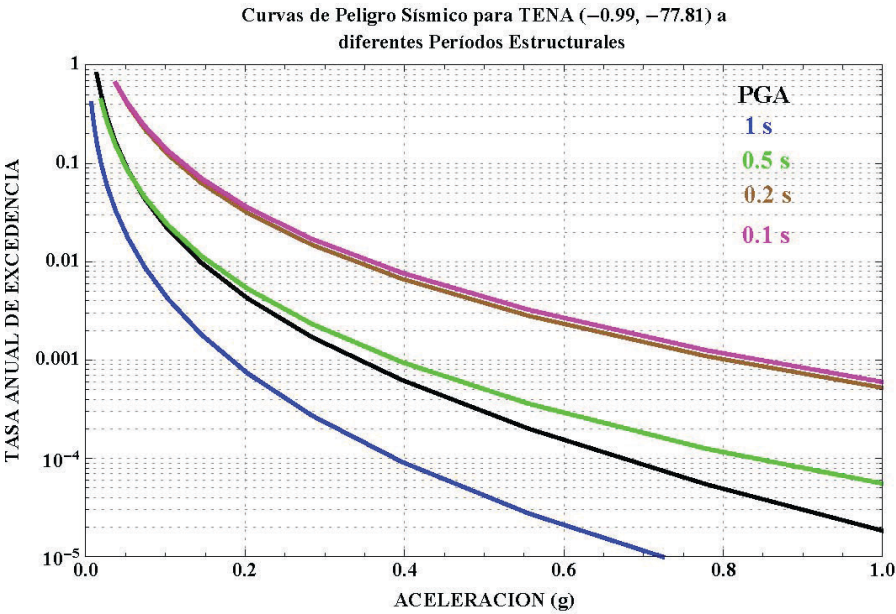
Figura 28 : Curvas de peligro sísmico, Tena.
