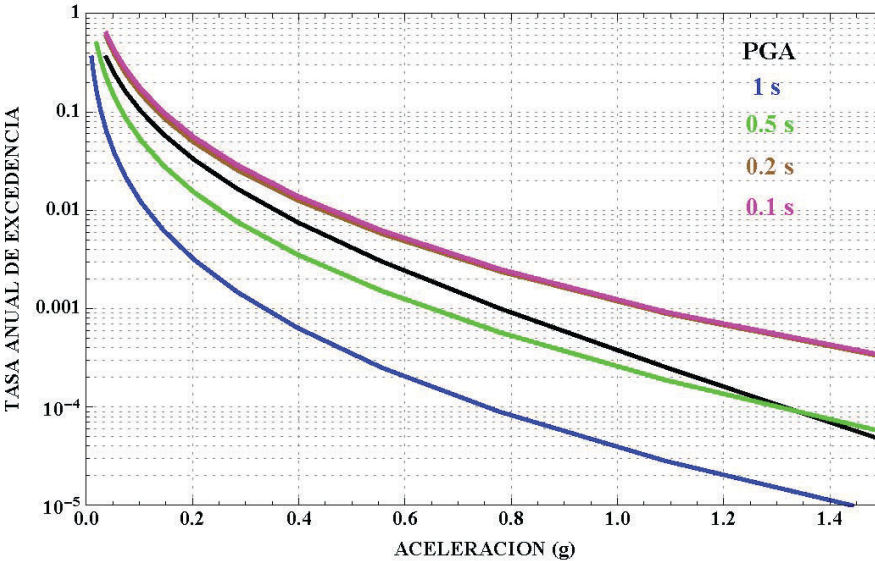
Curvas de Peligro Sísmico para PORTOVIEJO (-1.06; -80.46) a diferentes Periodos Estructurales
