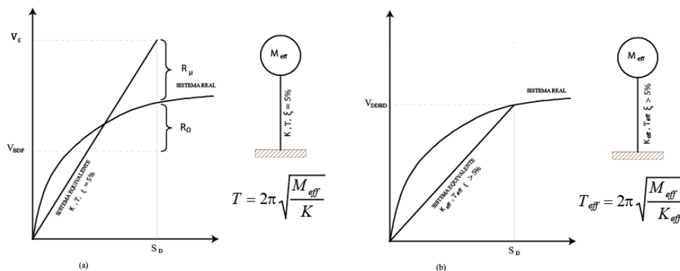
Figura 5 : Linearización equivalente
