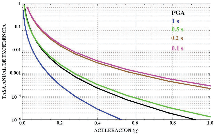
Figura 19 : Curvas de peligro sísmico, Loja.
