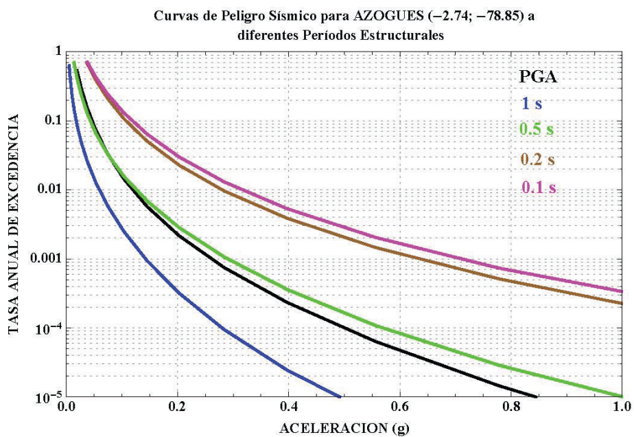
Figura 17 : Curvas de peligro sísmico, Azogues.
