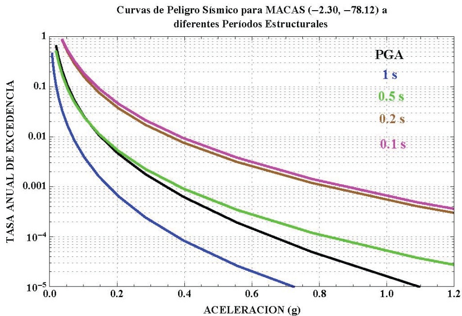
Figura 30: Curvas de peligro sísmico, Macas.
