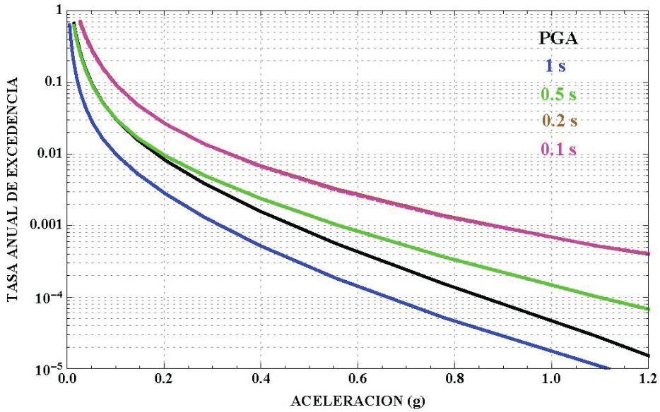
Figura 23: Curvas de peligro sísmico, Santo Domingo.
