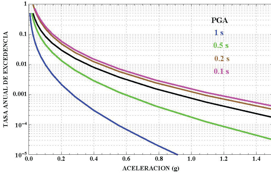
Figura 22: Curvas de peligro sísmico, Santa Elena
